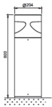
B: 50.7004.X双面出光灯具尺寸图
