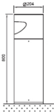
A: 50.7004.V单面出光灯具尺寸图
